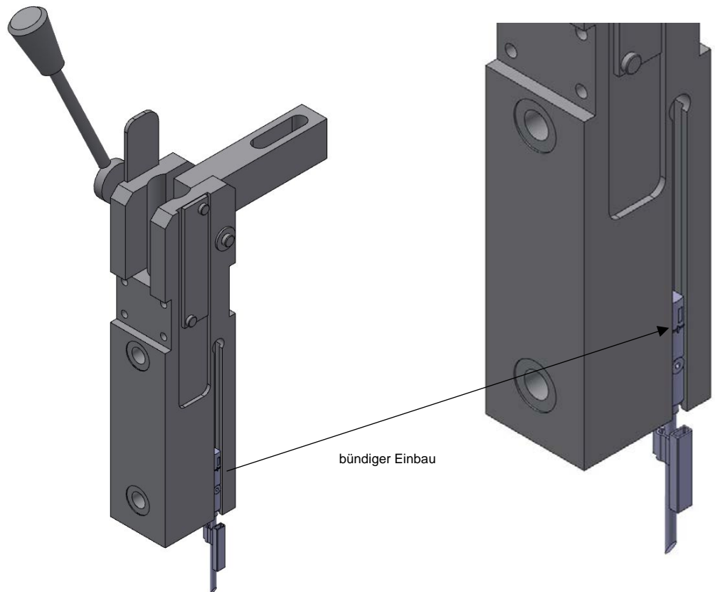
Beispiel: Spanner mit Endlagensensor
